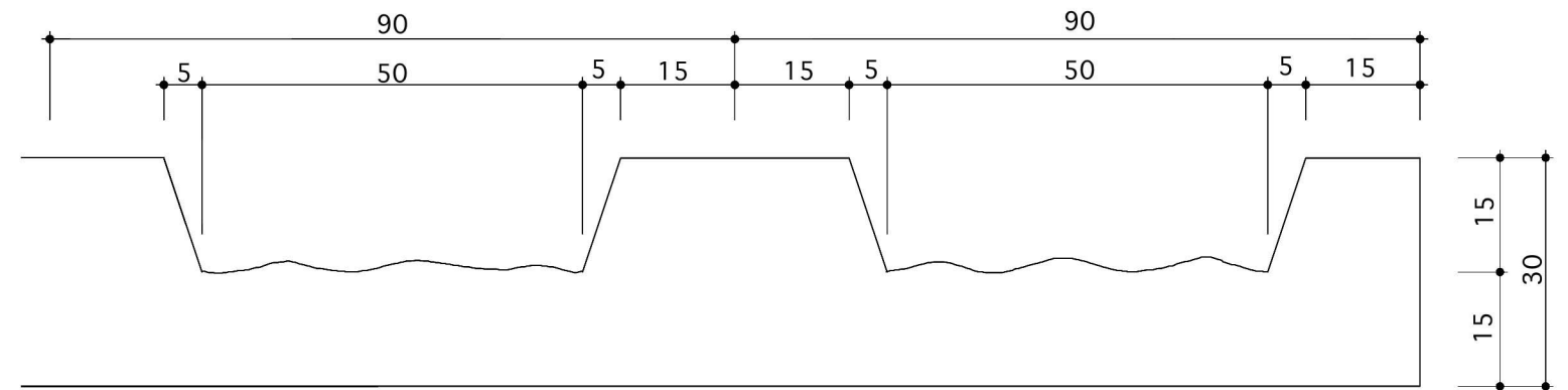
横拡大断面図 S=1/1
